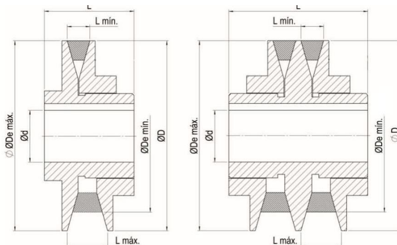
POLIAS REGULÁVEIS DE 1 CANAL
